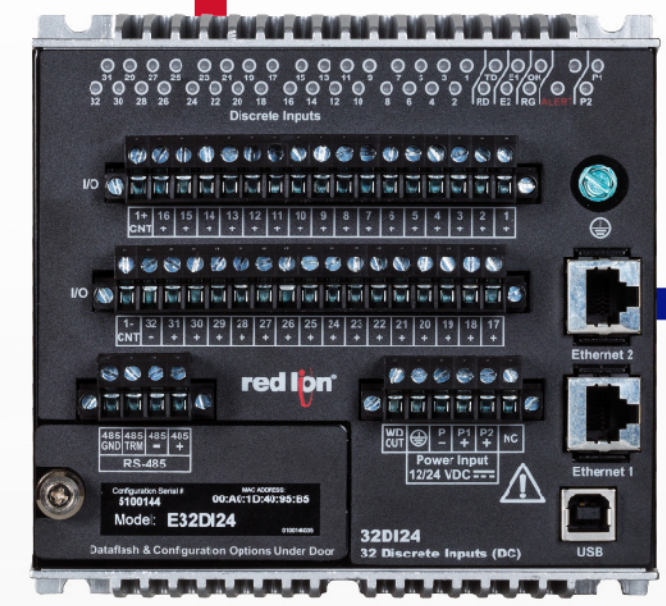
E3 I/O™ Module High-Density I/O Module
